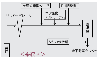
薬注装置(次亜塩素酸ソーダ)
